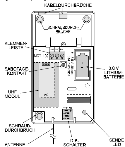
Abbildung 1: MCT-100 Innenansicht
