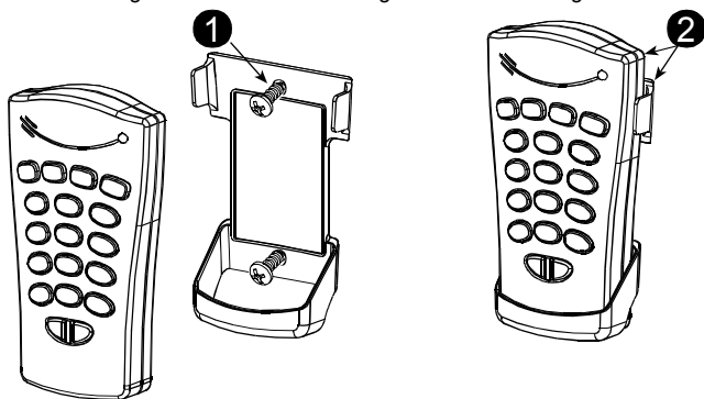
Abb. 2 - Montage
