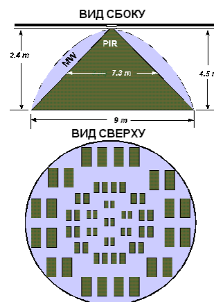
Рисунок 1. Зона обнаружения детектора DUO-24
