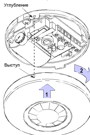
Рисунок 6. Установка крышки
